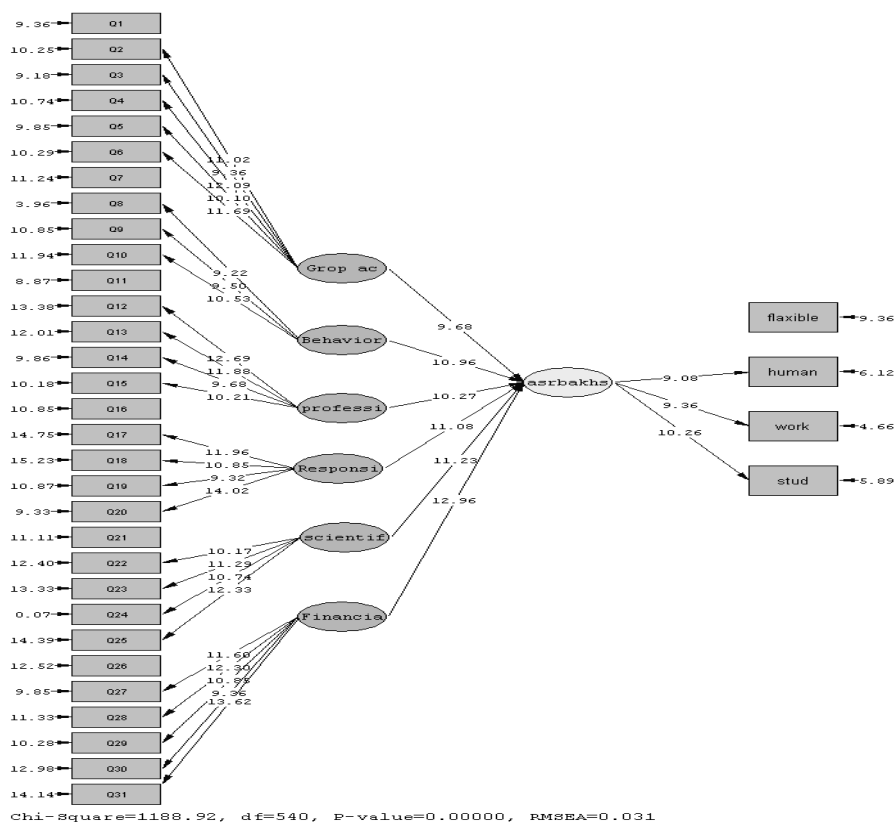
نمودار مسیر مدل ساختاری در حالت اعداد معناداری
