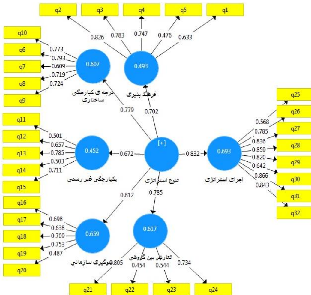
شکل ۳. ضرایب مسیر
