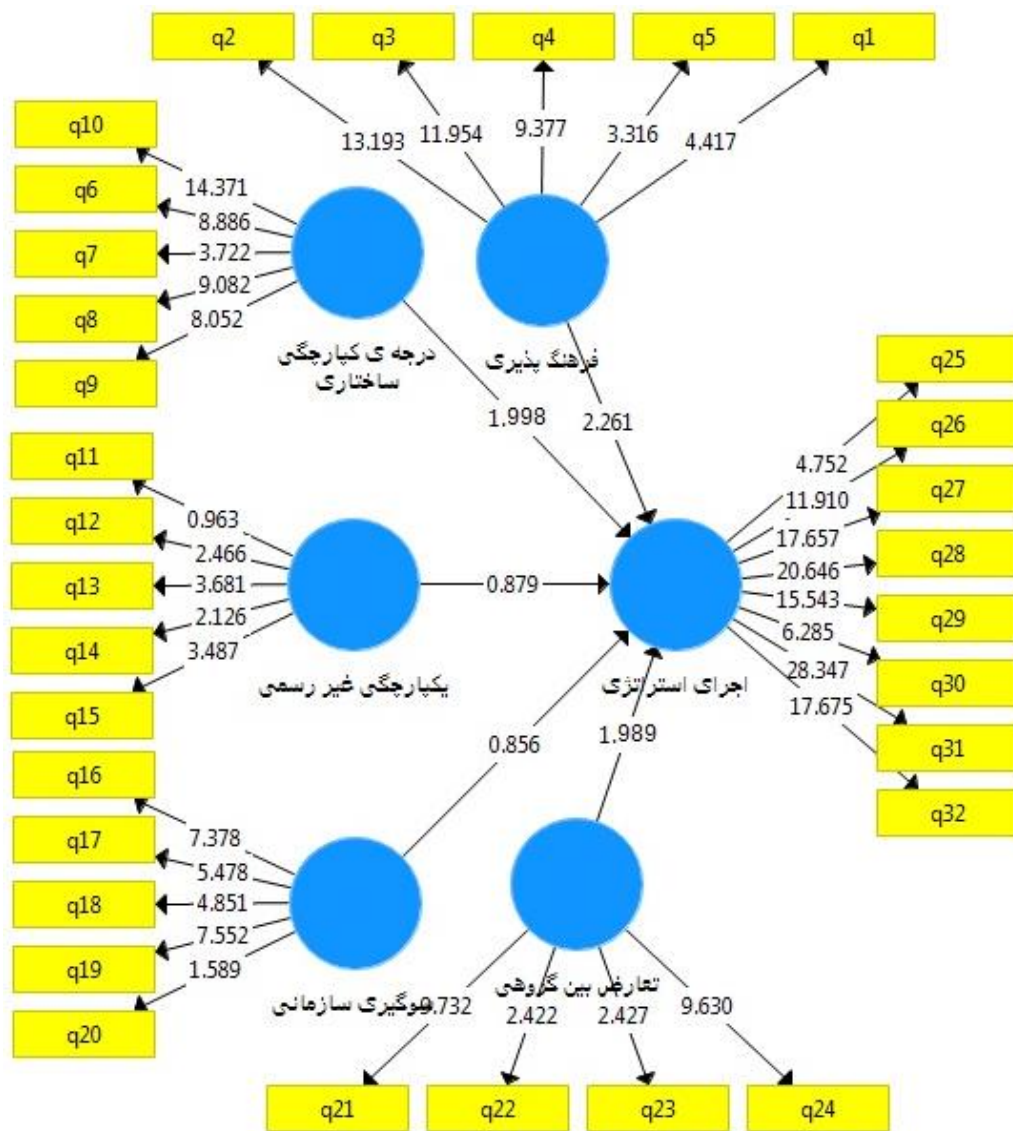
شکل ۶. ضرایب معناداری
