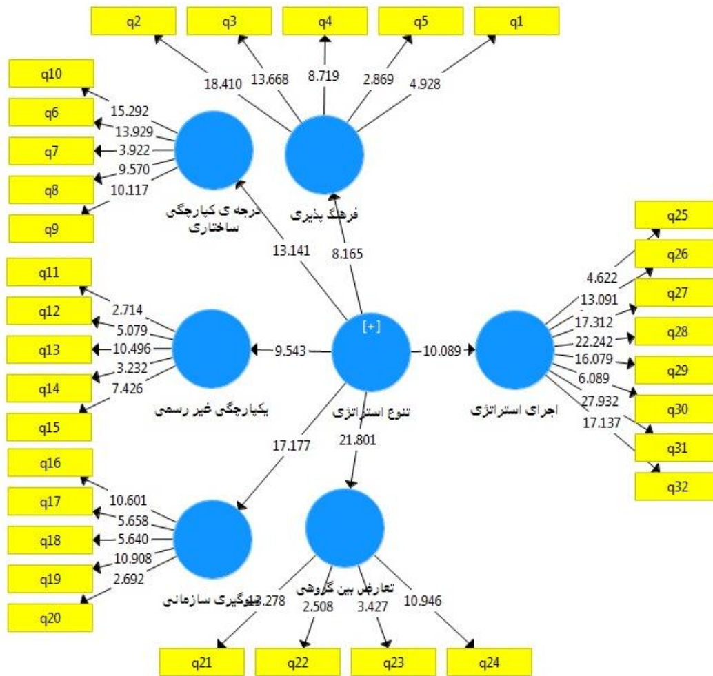
شکل ۴. ضرایب معناداری
